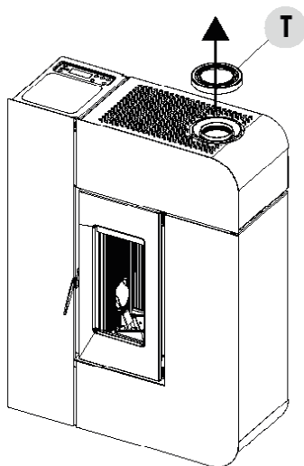
INSTALLAZIONE TIPO "COAX" USCITA FUMI DOPPIA PARETE
