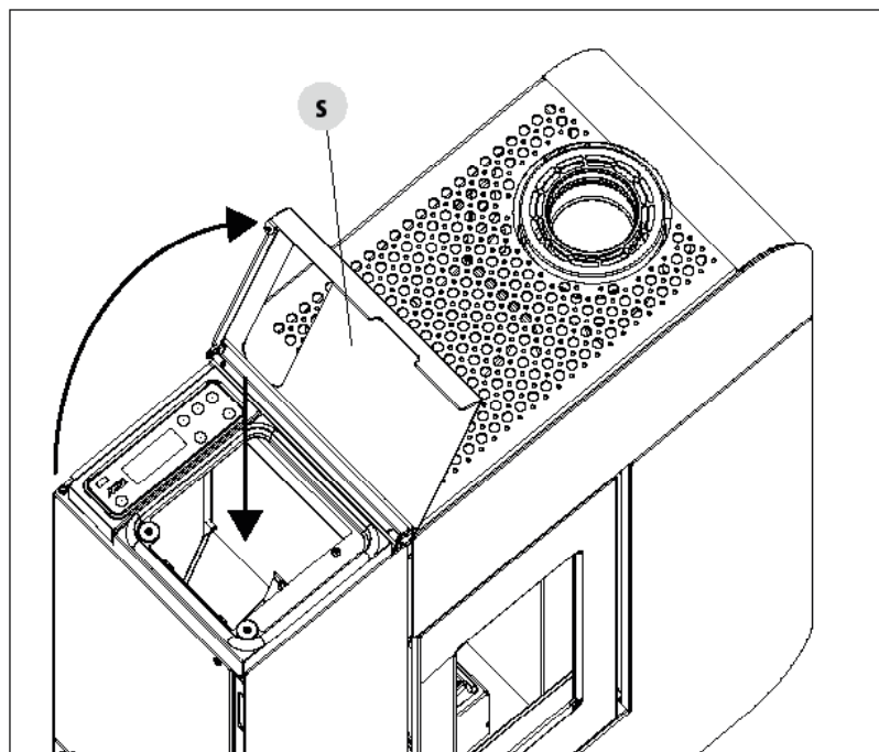
CHARGEMENT DES PELLETS
