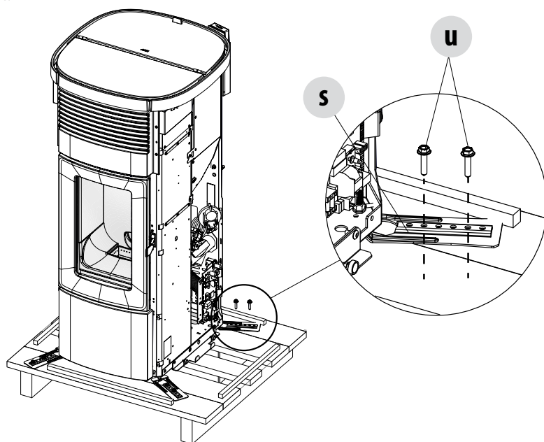
RETRAIT DES ÉTRIERS DE FIXATION POÊLES MUSA
