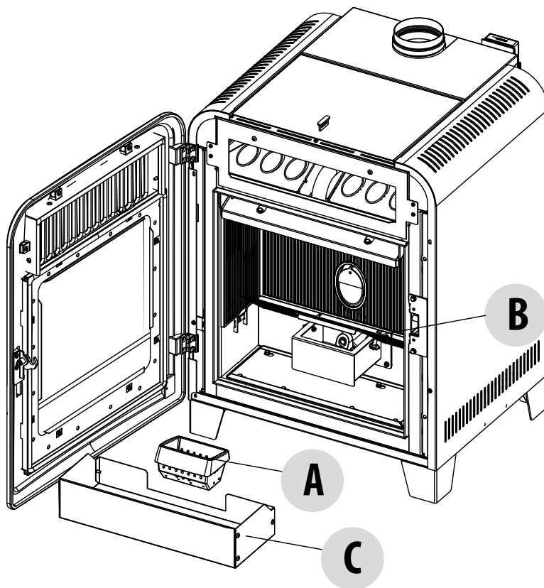
NETTOYAGE DU COMPARTIMENT INFÉRIEUR
