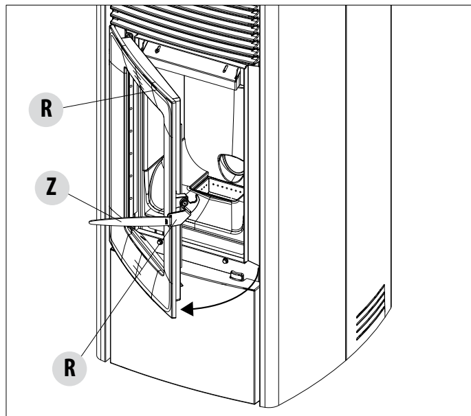
PORTE DU FOYER
