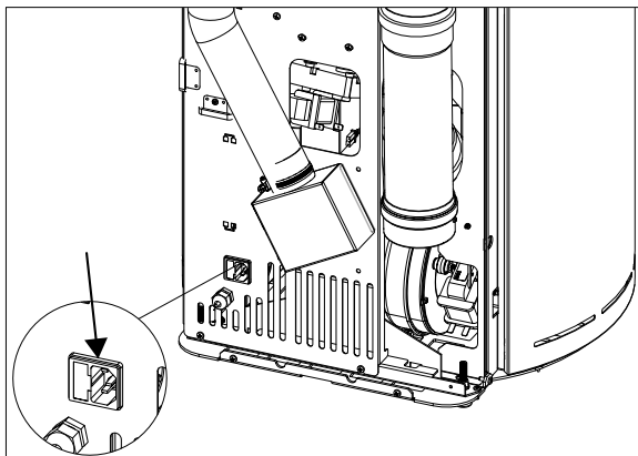
BRANCHEMENT ÉLECTRIQUE DU POÊLE
